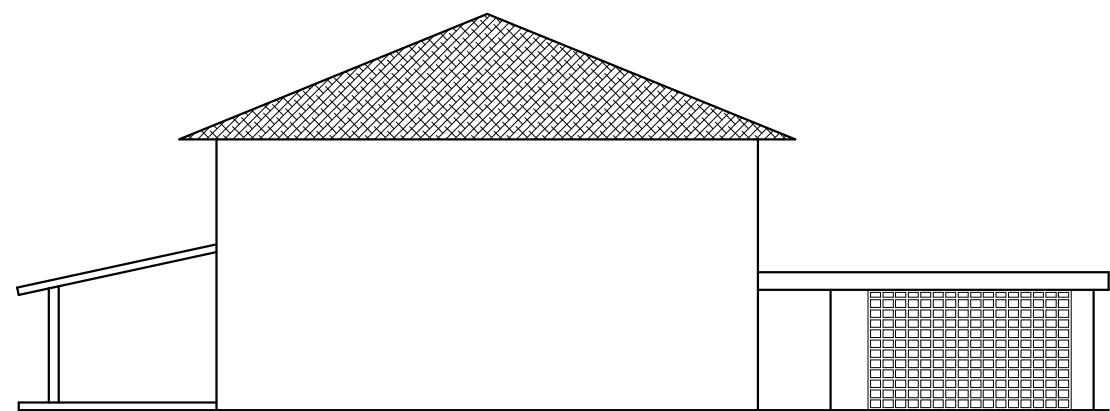
ELEVACAO OESTE - LATERAL
