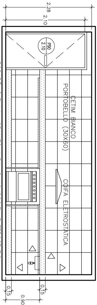
VISTA A
