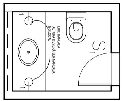
LAVABO 02 ARANDELAS METÁLICAS VIBRO (8W) LED 2700K MODELO PÍCOLO W LED - MARCA LUMINI - COR ALUMINIO ESCURIDO COLOCAÇÃO DE ESPELHO LAMPIDADO COLADO SOBRE A BANCADA ESP 5mm (1,40 X 0,90) m
