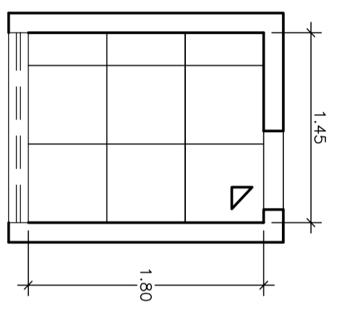
LAVABO VISTA B PISO (60 X 60) E SOLTEIRA GRANITO BRANCO SÃO PAULO PAGINAÇÃO PISO 1/20
