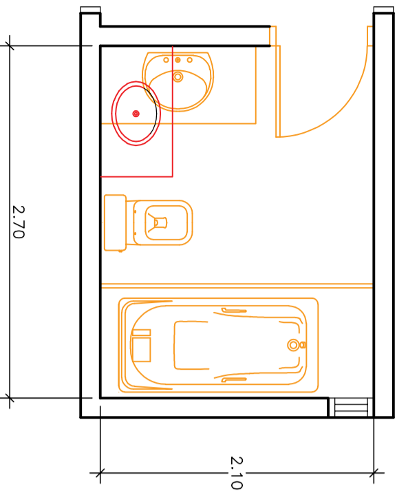
PLANTA EXISTENTE 1/25
