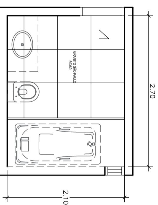
PAGINAÇÃO PISO 1/25
