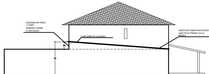
ELEVACAO OESTE - LATERAL 1/75
