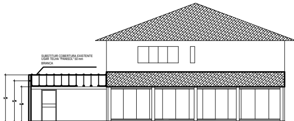
ELEVACAO NORTE - AREA VERDE 1/75
