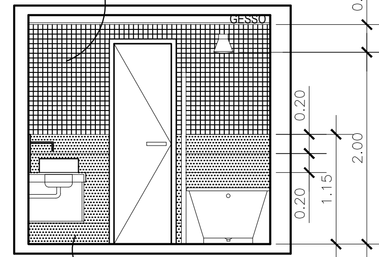
VISTA-B 1/20 PISO, RODAPÉ, 1/2 PAREDE, BANCADA EM GRANITO BRANCO SÃO PAULO
