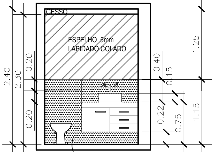
VISTA-A 1/20 PISO, RODAPÉ, 1/2 PAREDE, BANCADA EM GRANITO BRANCO SÃO PAULO
