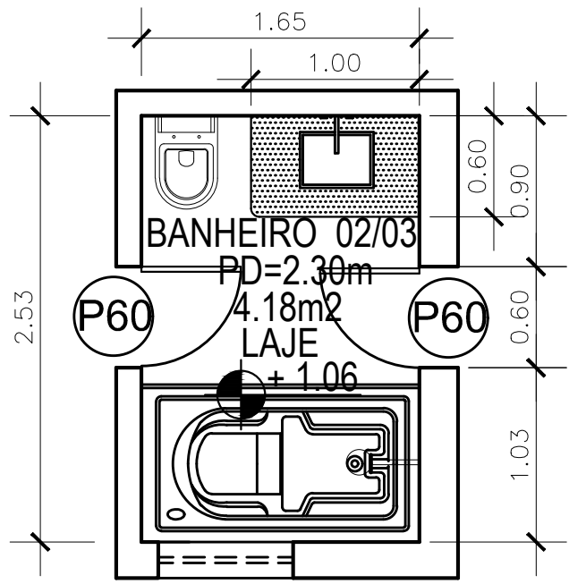
PLANTA-BAIXA 1/20
