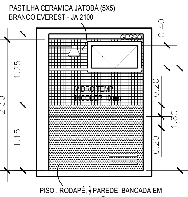
VISTA-C 1/20 PISO, RODAPÉ, 1/2 PAREDE, BANCADA EM GRANITO BRANCO SÃO PAULO
