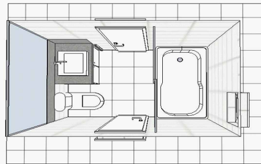
BANHEIRO 02/03 S/ESC
